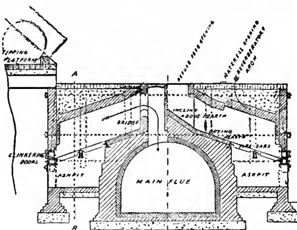
FIG. 1.—Fryer's Destructor.
